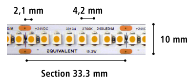
Section 33,3 mm
