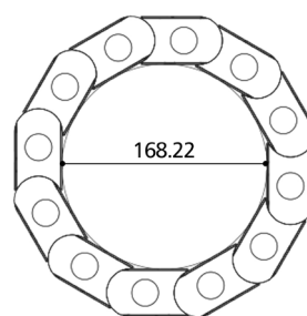
DIAMÈTRE DE COURBURE MINIMUM
