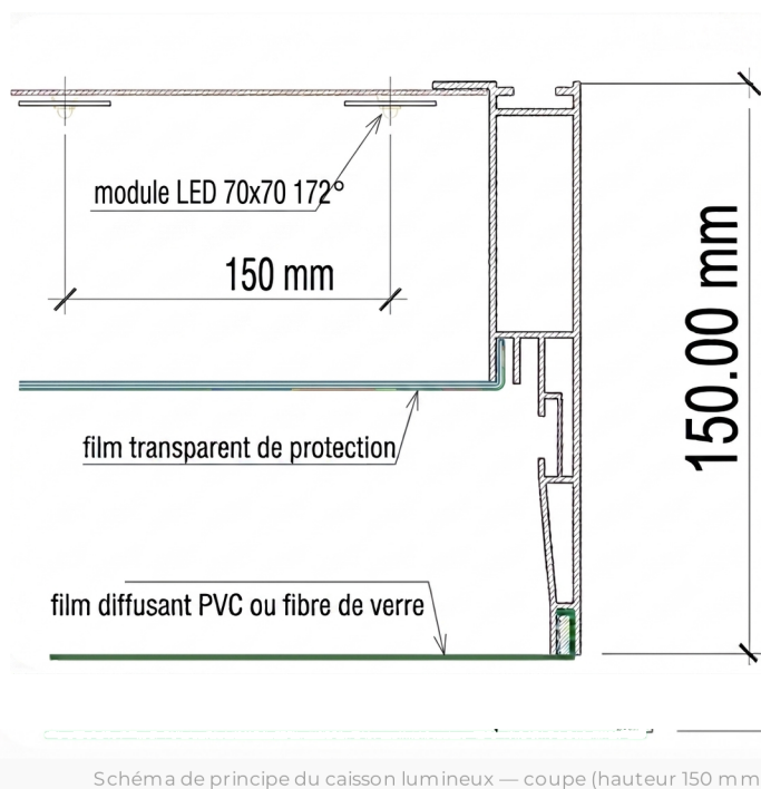
Schéma de principe du caisson lumineux — coupe (hauteur 150 mm)
